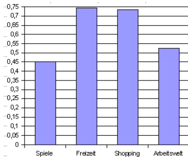
Abbildung 11: Precision Wert von del.icio.us getrennt nach Themengebieten
